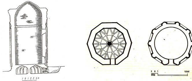
Şəkil 15. Türbənin kəsiyi, sərdabə və gövdəsinin planı.
