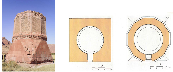
Şəkil 17. Gülüstan türbəsi, sərdabə və gövdəsinin planı.
