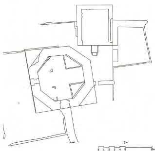
Şəkil 7. Xarabagilan türbələrinin baş planı və türbələrin qalıqları.
