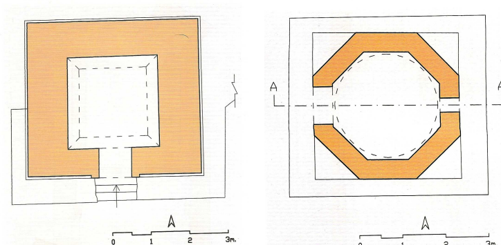
Şəkil 6. XII əsrdə tikilmiş 1-ci türbənin sərdabə və gövdəsinin planı.
