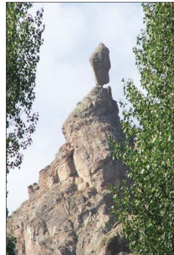
"Gəlinqaya (Gəlinədaş)" - Ordubad rayonunun Unus və Pəzməri kəndlərini birləşdirən yoldan yuxarıda yerləşən və qadın siluetini xatırladan Orta Eosenin vulkanogen süxurlarından təşkil olunmuş ekzotik qaya.
